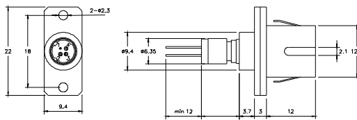
SC Receptacle
