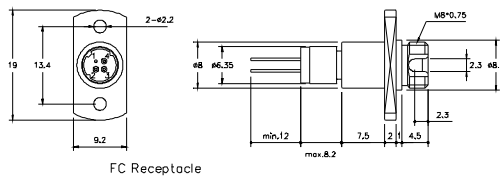
FC Receptacle
